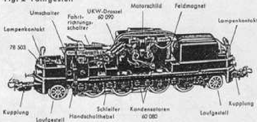
Fig. 2 Fahrgestell
