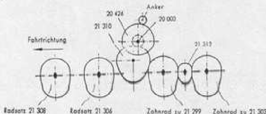
Fig. 4 Anordnung der Getrieberäder
