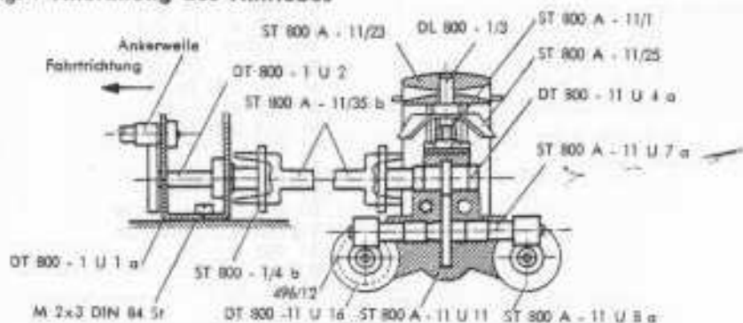
Fig. 4 Anordnung des Antriebes
