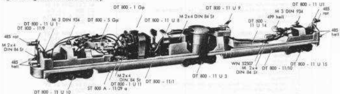
Fig. 2 Fahrgestell DT 800 - 11 Gp
