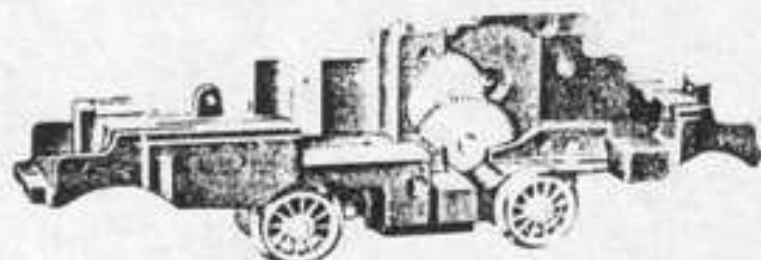
Fig. 3 Treibgestell
