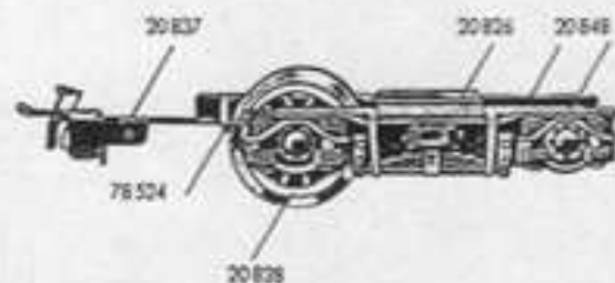
Fig. 6 Laufgestell
