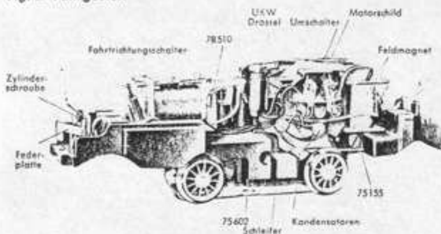
Fig. 2 Fahrgestell
