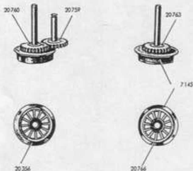
Fig. 6 Laufgestell
